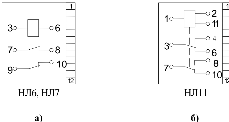
Рисунок 3 – Схемы подключения реле
